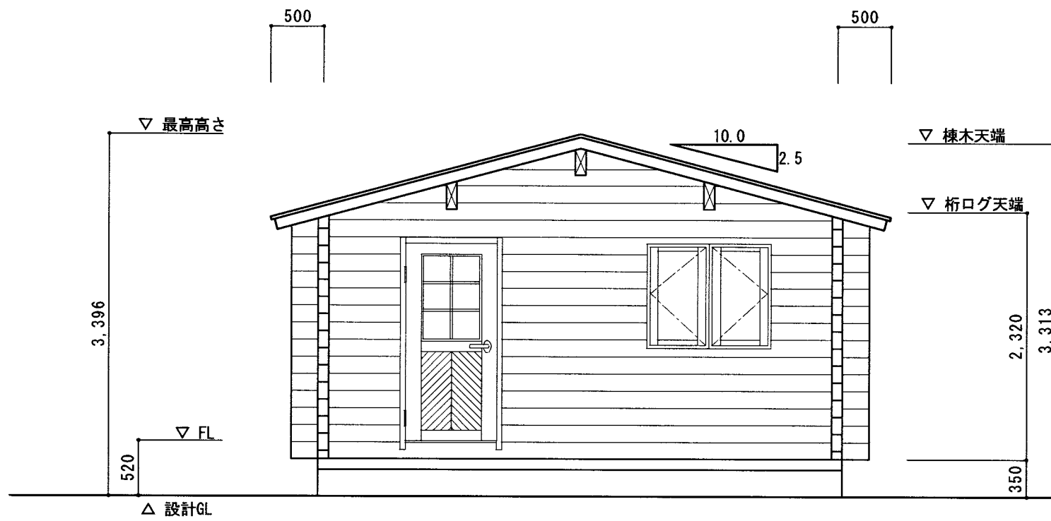
立面図 S=1/50
