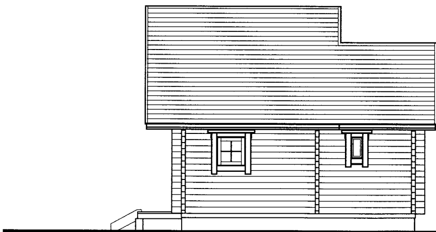
東側立面図 1:100
