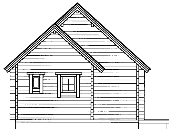
北側立面図 1:100
